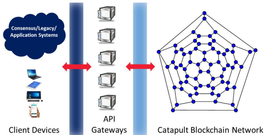
【図3】他のシステム、あるいはクライアントの端末と接続するためのAPIゲートウェイを用いたアーキテクチャ。現行の標準と齟齬をきたさない。
