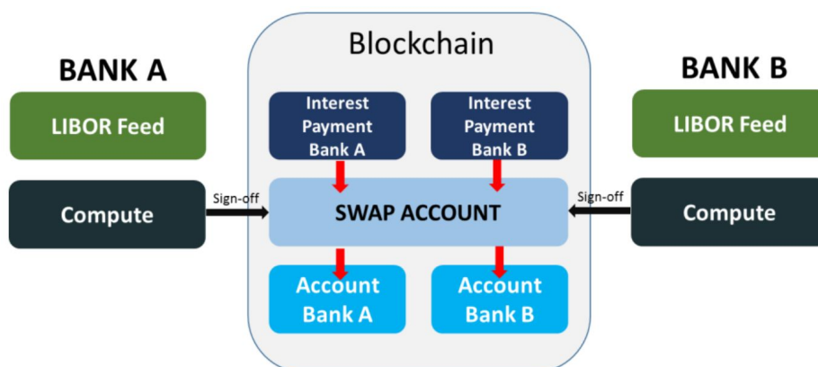
【図6】 ブロックチェーン上での金利スワッピング
